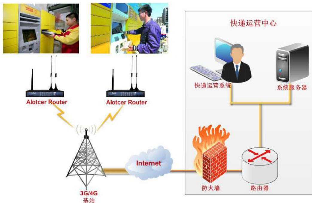
ROUTER 应用拓扑图
